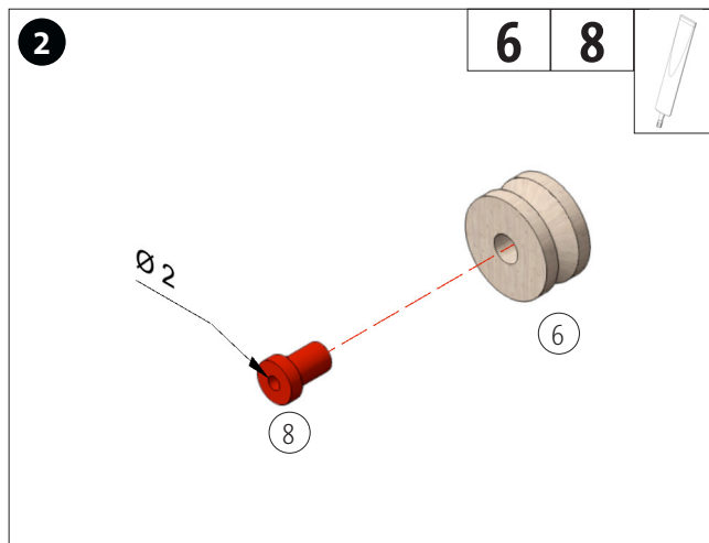
Reduzierstück (8, Ø2mm) in ein Schnurlaufrad (6) kleben
