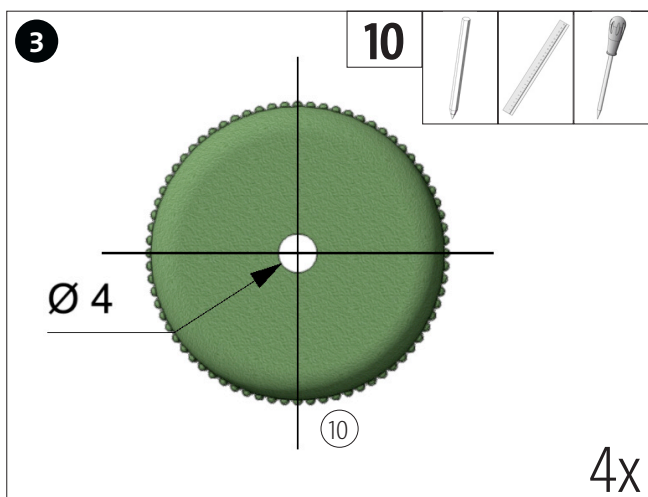
Flaschendeckel säubern und mittig ein Loch mit etwa Ø4mm einstechen.
