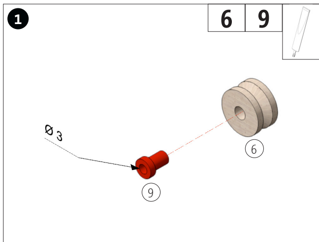
Reduzierstück (9, Ø3mm) in ein Schnurlaufrad (6) kleben
