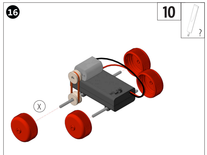
Die 4 vorbereiteten Räder auf die Achsen stecken, bei Bedarf festkleben.
