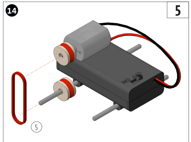
Den Gummiring (5) doppelt legen, mehrmals zwischen den Fingern dehnen, damit dieser nicht zu stramm sitzt, und in die Lauffläche einlegen.
