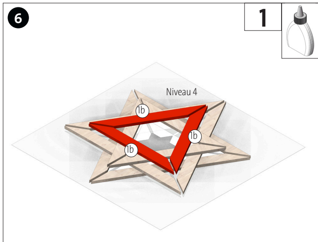
Niveau 4 van drie houten latten (1b) volgens het sjabloon verlijmen.
