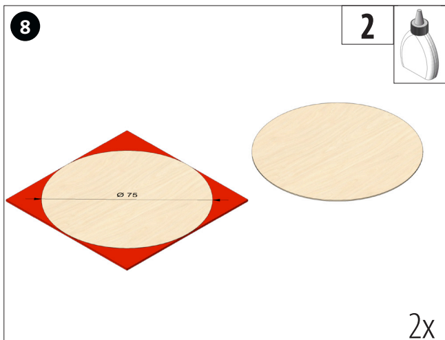
Uit de beide houtfineer stukken elk een cirkel van \varnothing 75 mm snijden.
