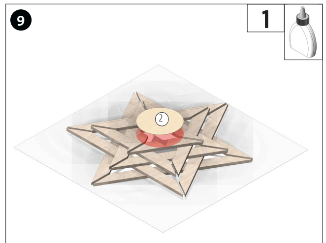
Een houtfineer cirkel (2) gecentreerd op niveau 5 lijmen.
