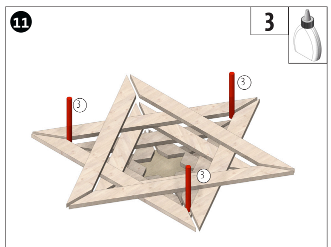
Die Rundstäbe (3), wie gezeigt einleimen.
