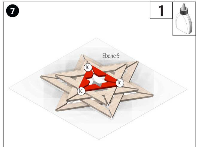
Ebene 5 aus drei Holzleisten (1c) nach Schablone aufleimen.
