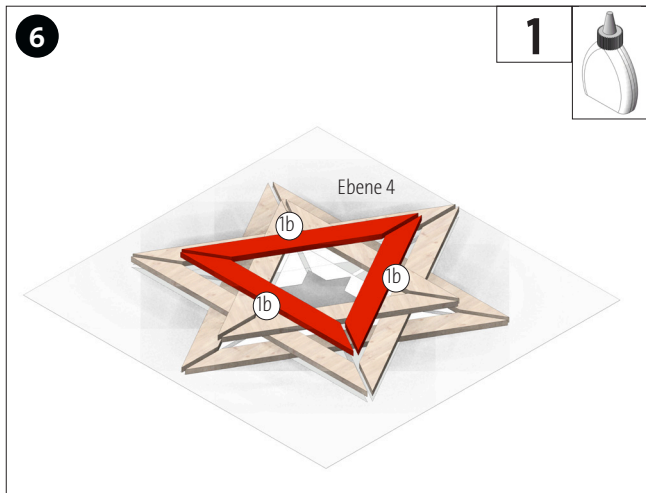
Ebene 4 aus weiteren drei Holzleisten (1b) nach Schablone aufleimen.
