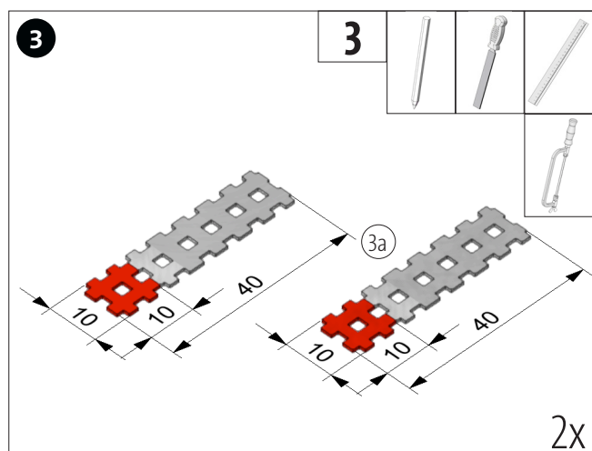
Cortar 2 trozos de tira perforada (3) de 40 mm y desbarbar los bordes. Marcar la línea a doblar en cada lado.
