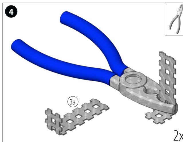
Doblar las dos tiras perforadas (3a) con el alicate para que formen un ángulo de 90°.
