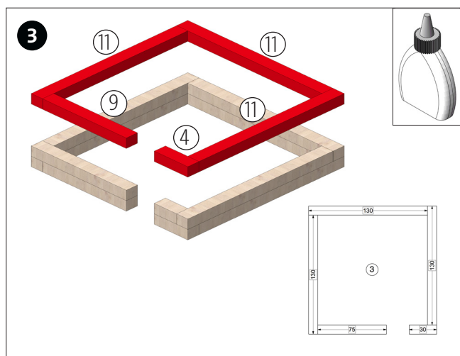
Die Ebene 3 zusammenleimen und auf Ebene 2 aufleimen. (s. Abb.)
