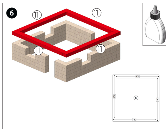
Die Ebene 6 zusammenleimen und auf Ebene 5 aufleimen. (s. Abb.)
