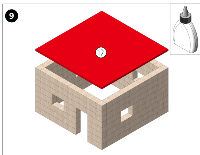
Deckplatte (12) wie abgebildet bündig auf Ebene 8 aufleimen.
