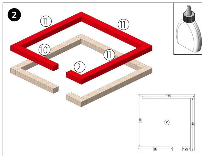
Die Ebene 2 zusammenleimen und auf Ebene 1 aufleimen. (s. Abb.)
