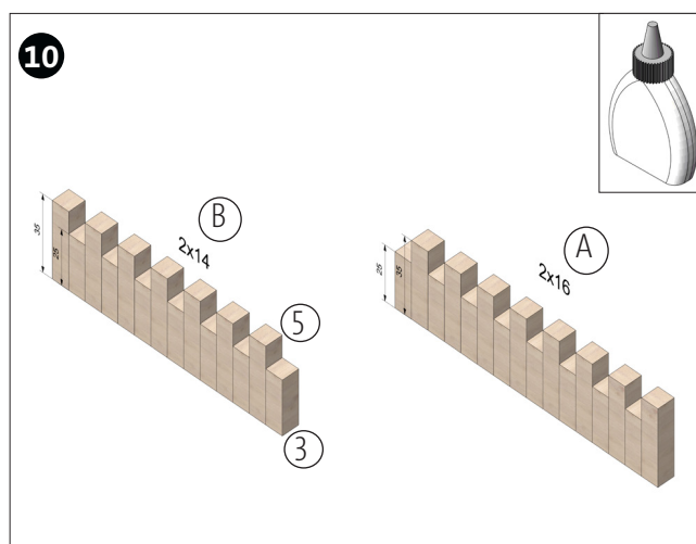
Wie abgebildet 2x 14 Leistenstücke (3+5) zusammenleimen. Ebenso 2x16 Leistenstücke (3+5) zusammenleimen. Bei allen 4 Zinnenleisten den Leim gut trocknen lassen.
