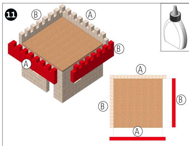
Die Zinnenleisten (A+B) wie abgebildet an der Ebene 8 anleimen.
