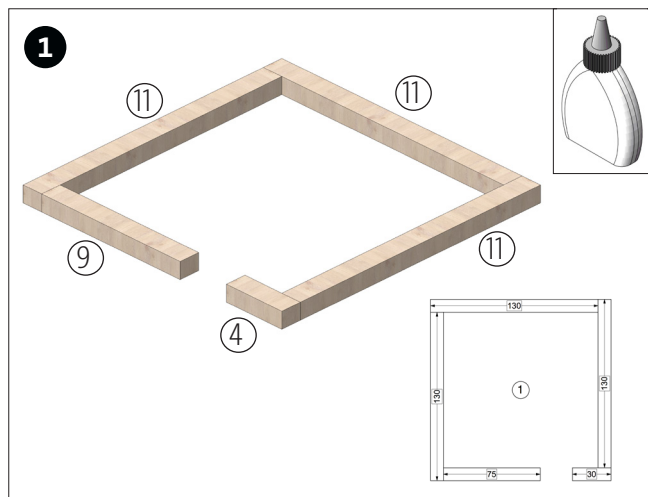
Die Ebene 1 des Hauses wie abgebildet zusammenleimen.
