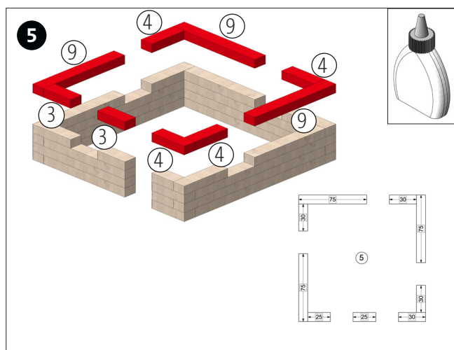
Die Ebene 5 zusammenleimen und auf Ebene 4 aufleimen. (s. Abb.)
