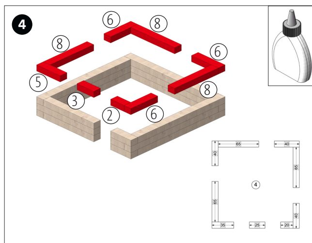
Die Ebene 4 zusammenleimen und auf Ebene 3 aufleimen. (s. Abb.)
