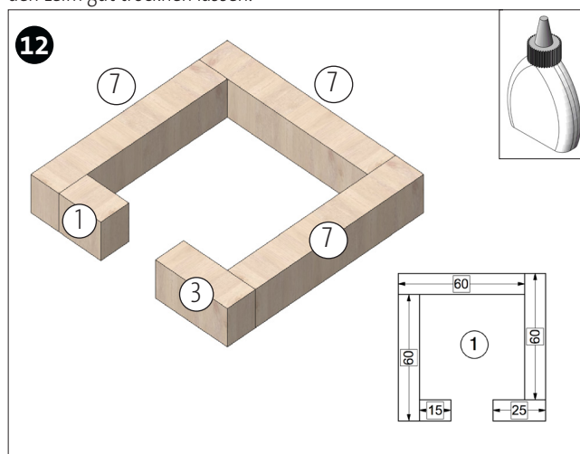
Die Ebene 1 des Turmes wie abgebildet zusammenleimen.
